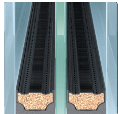
Warme Kante – thermisch optimierter Scheibenverbund \psi (Psi) bis 0,031 W/(m 2 K)
